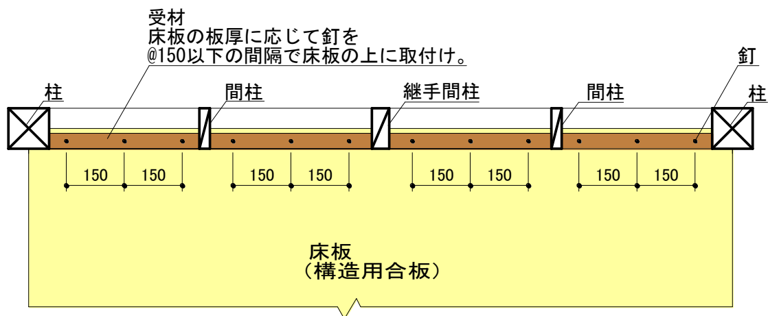
水平断面図
