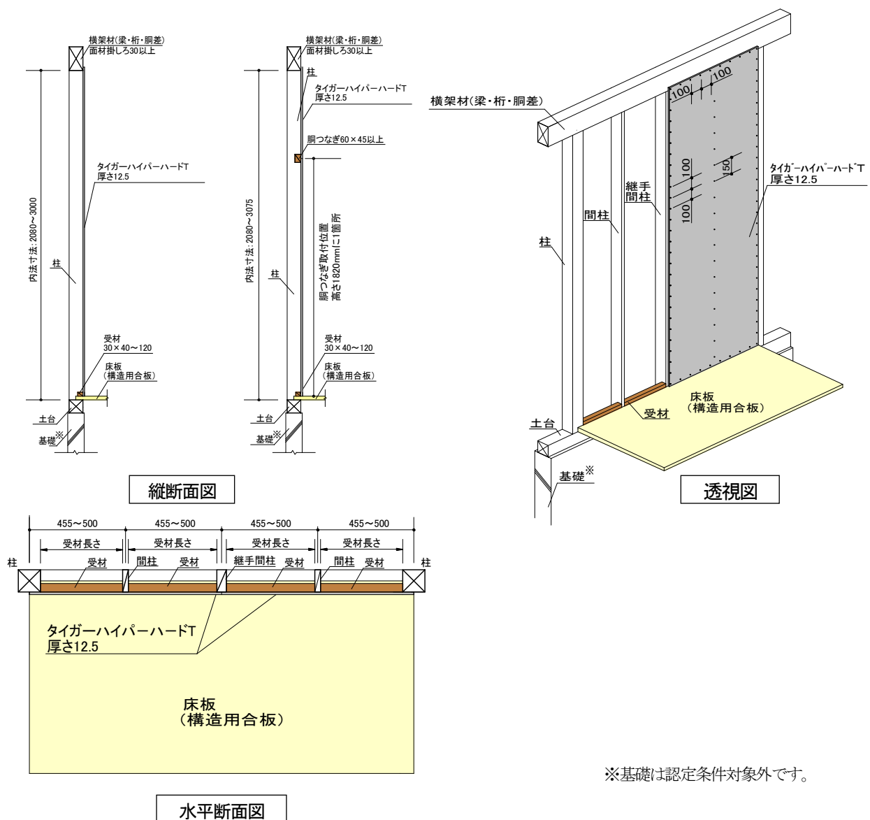
【木造軸組耐力壁（大壁造床勝ち仕様） 概要図 単位：m
